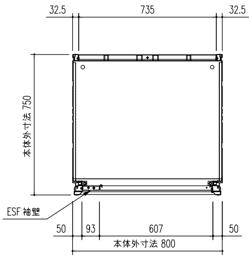
平面図 (S=1/20)
