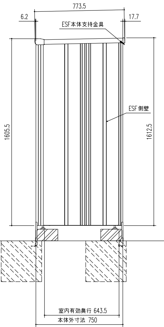
側面図 (S=1/20)
