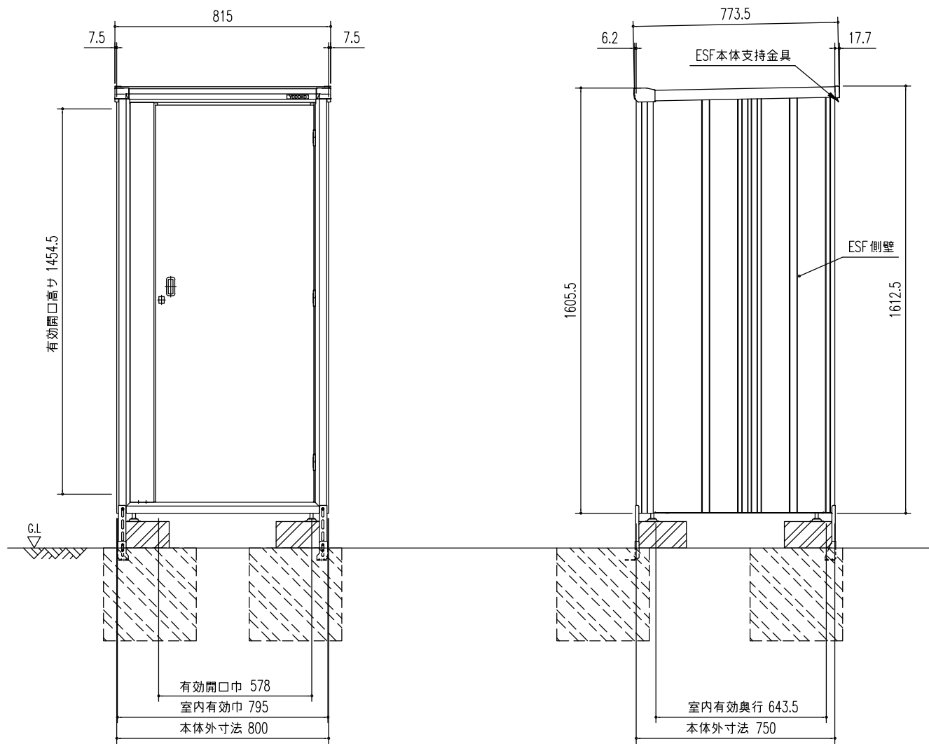
正面立面図 (S=1/20)
