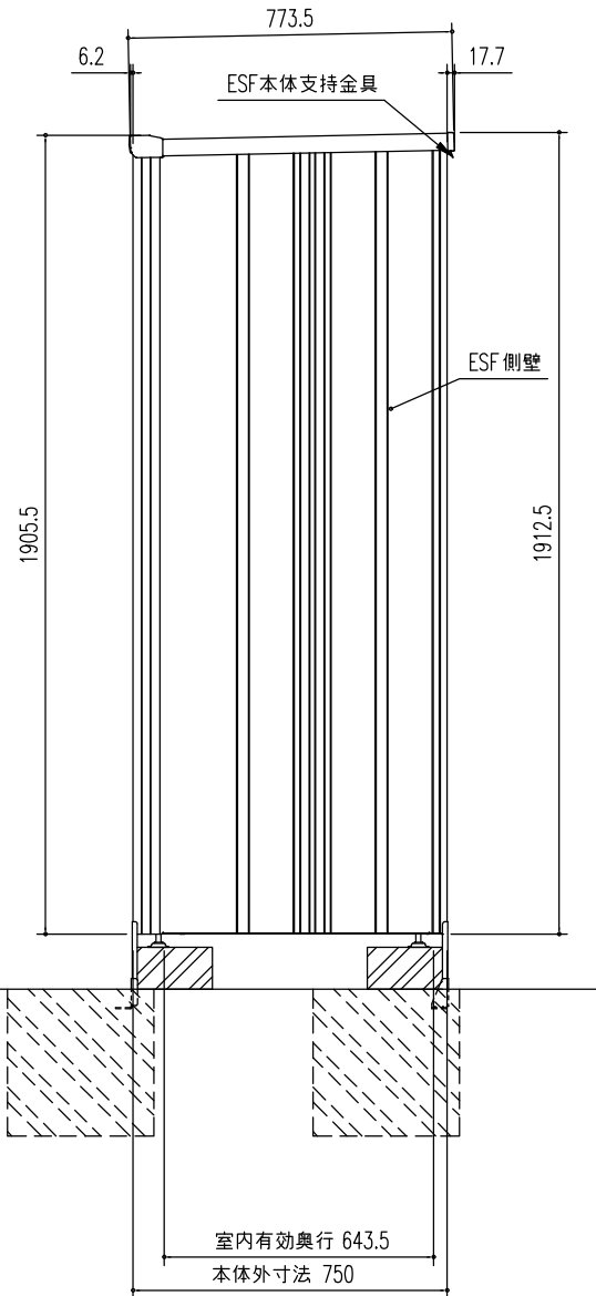
側面図 (S=1/20)
