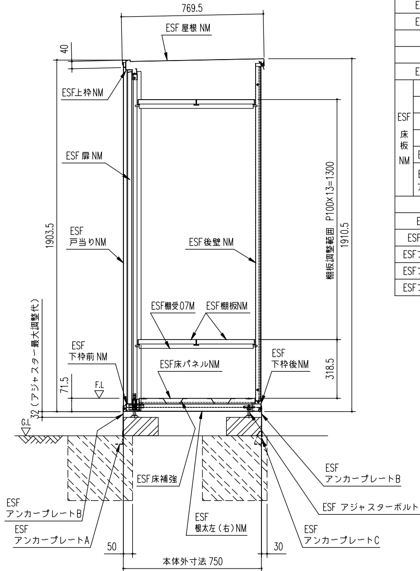
矩計図 (S=1/20)
