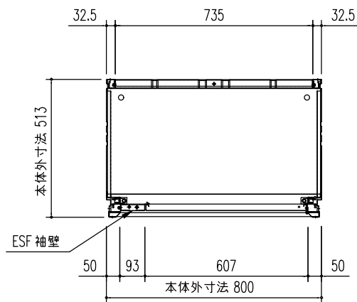
平面図 (S=1/20)
