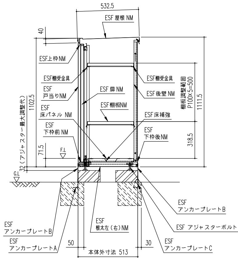
矩計図 (S=1/20)
