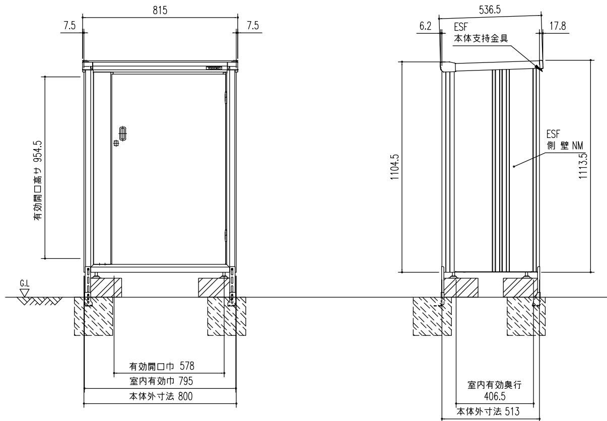
正面立面図 (S=1/20)
