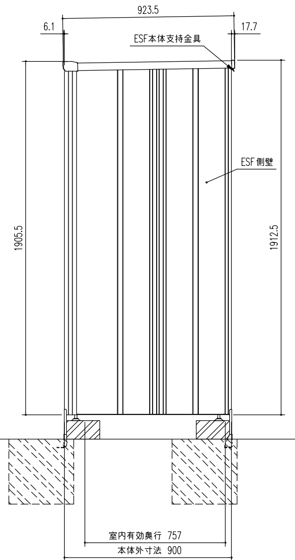
側面図 (S=1/20)
