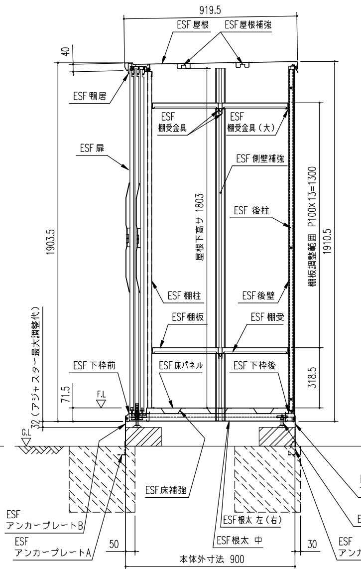
矩計図 (S=1/20)
