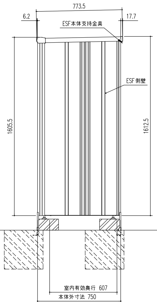
側面図 (S=1/20)
