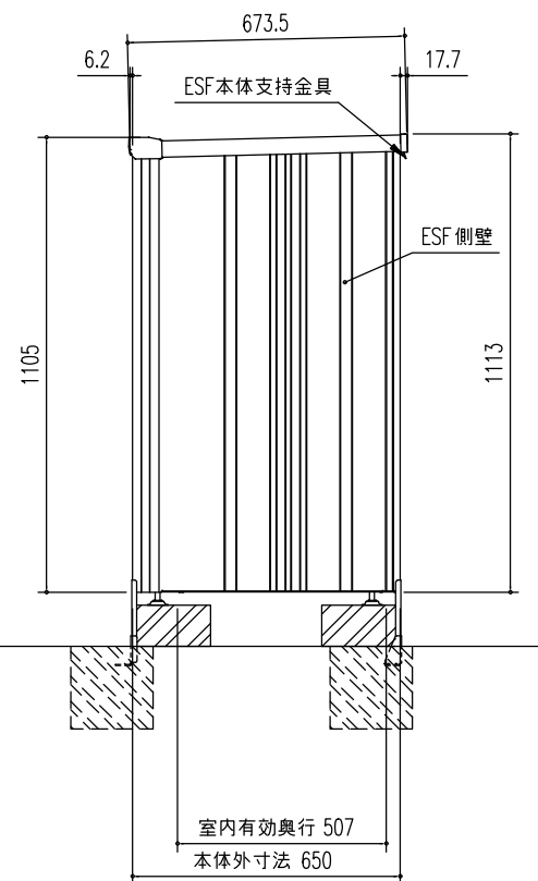
側面図 (S=1/20)
