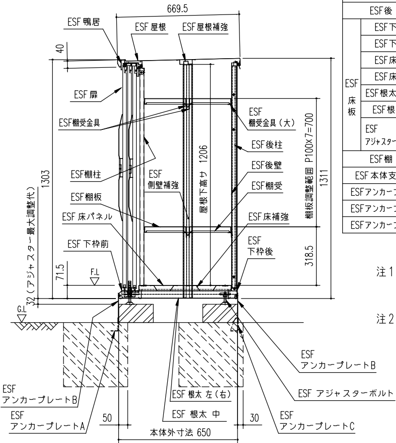
矩計図 (S=1/20)
