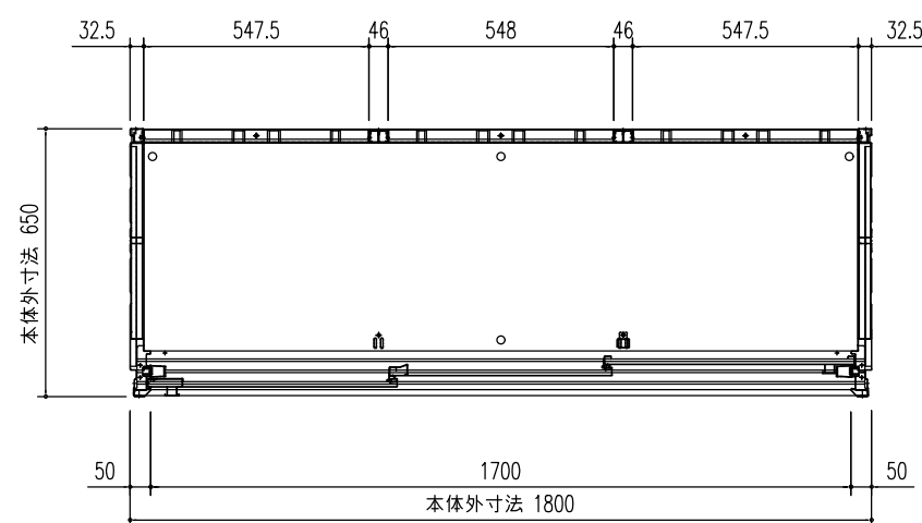
平面図 (S=1/20)
