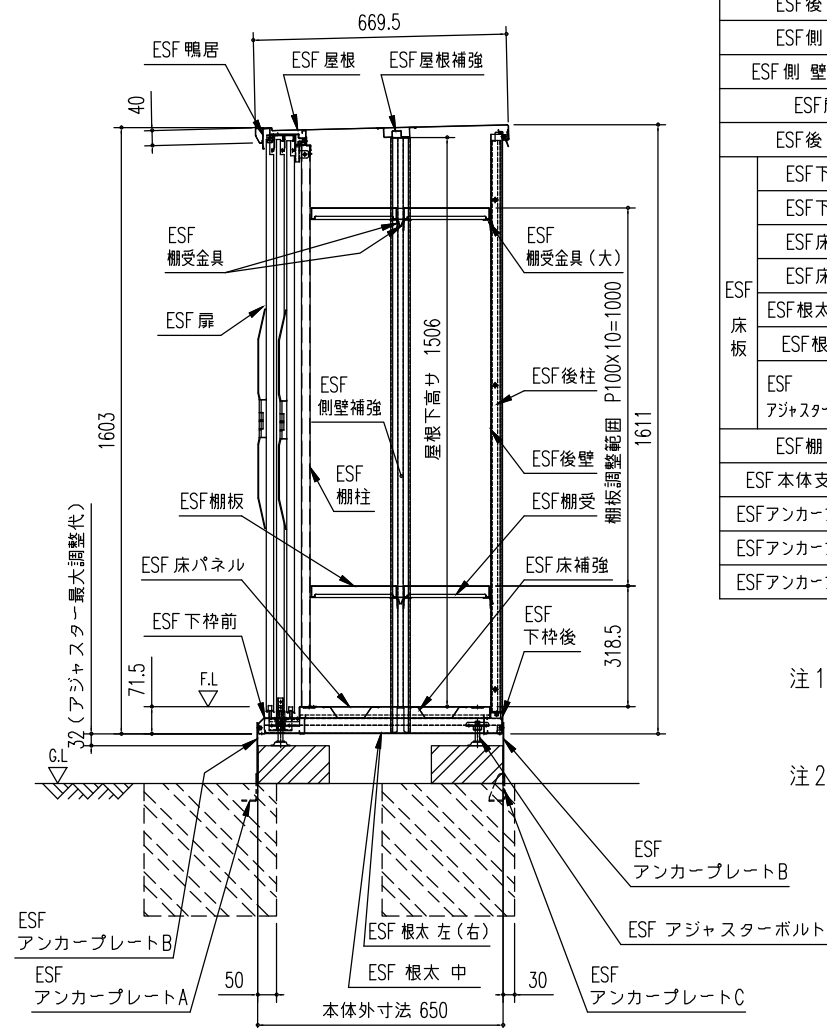
矩計図 (S=1/20)
