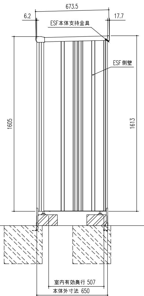
側面図 (S=1/20)
