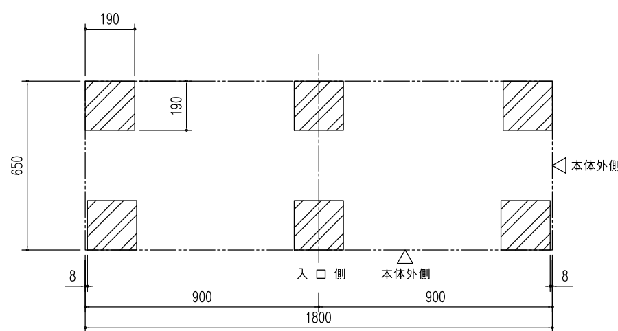
ブロック基礎伏図 (S=1/20)
