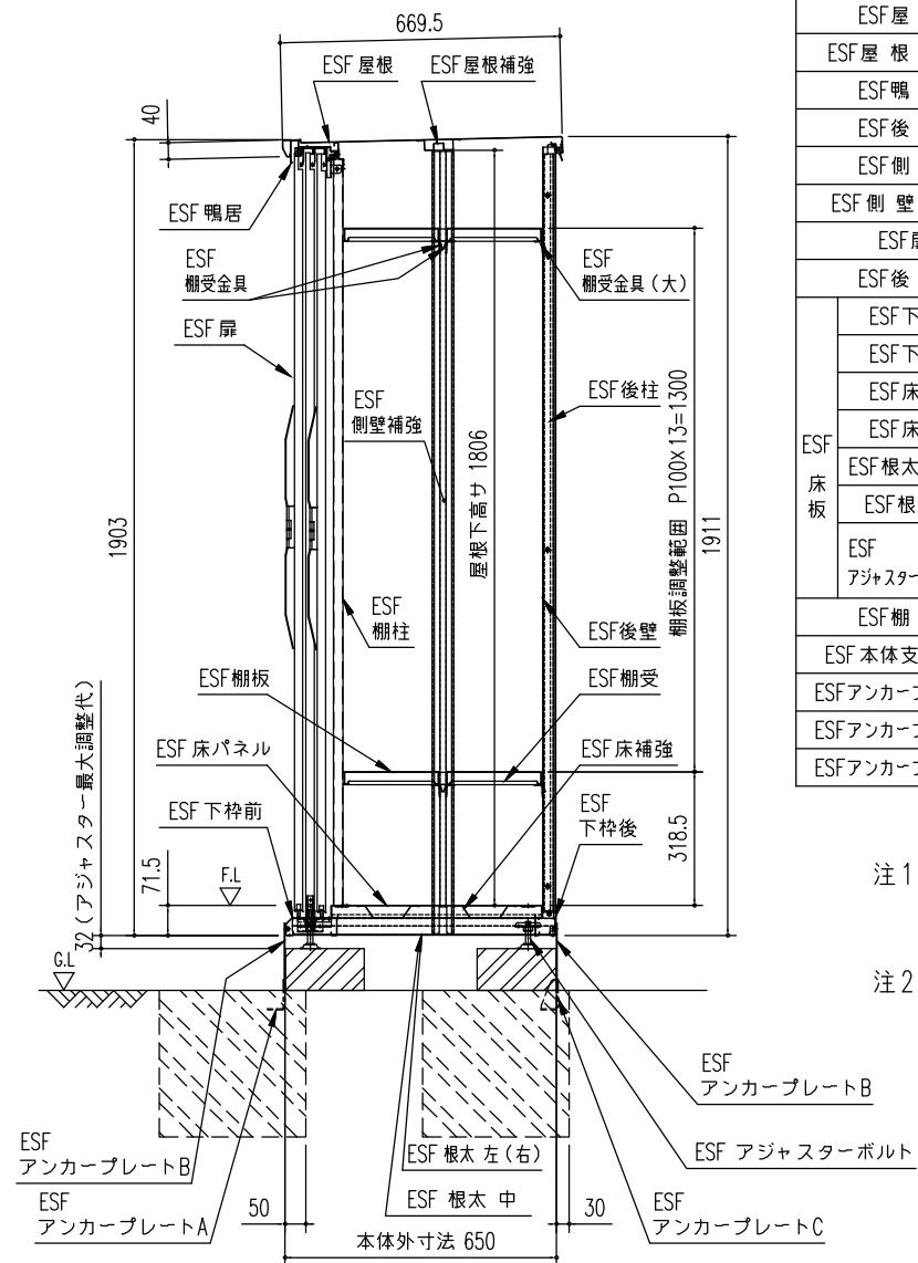
矩計図 (S=1/20)
