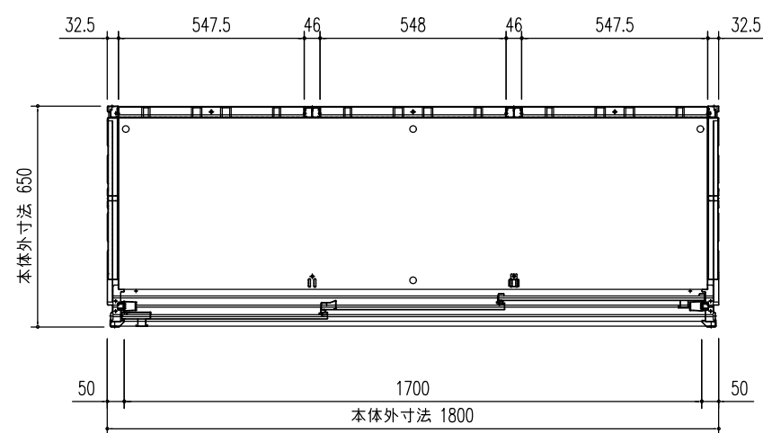
平面図 (S=1/20)
