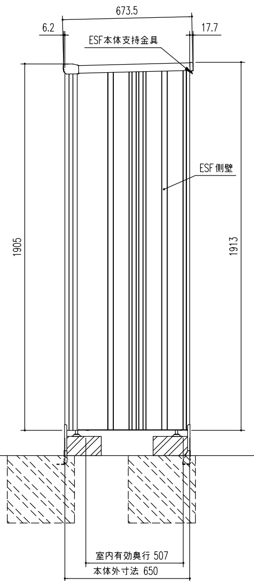
側面図 (S=1/20)
