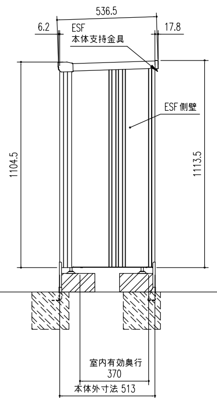
側面図 (S=1/20)
