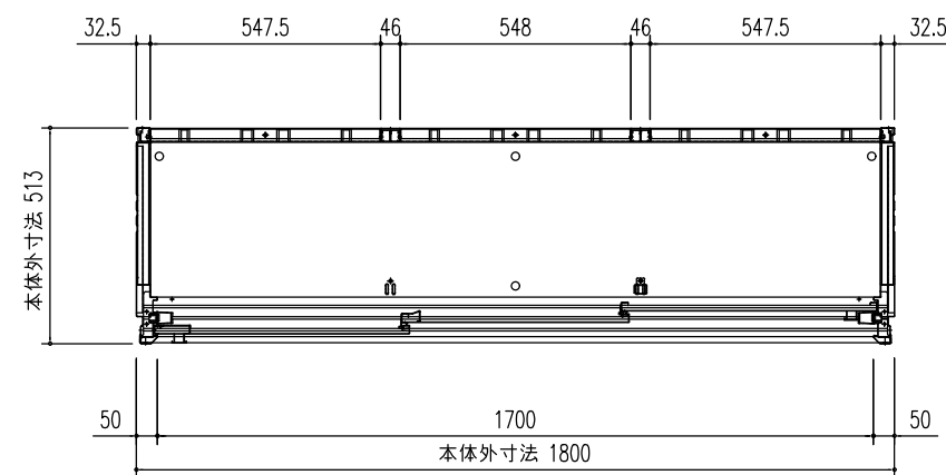
平面図 (S=1/20)
