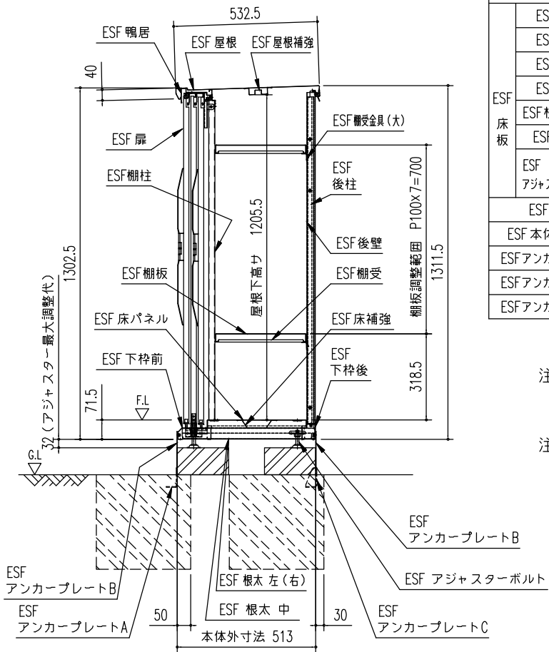
矩計図 (S=1/20)
