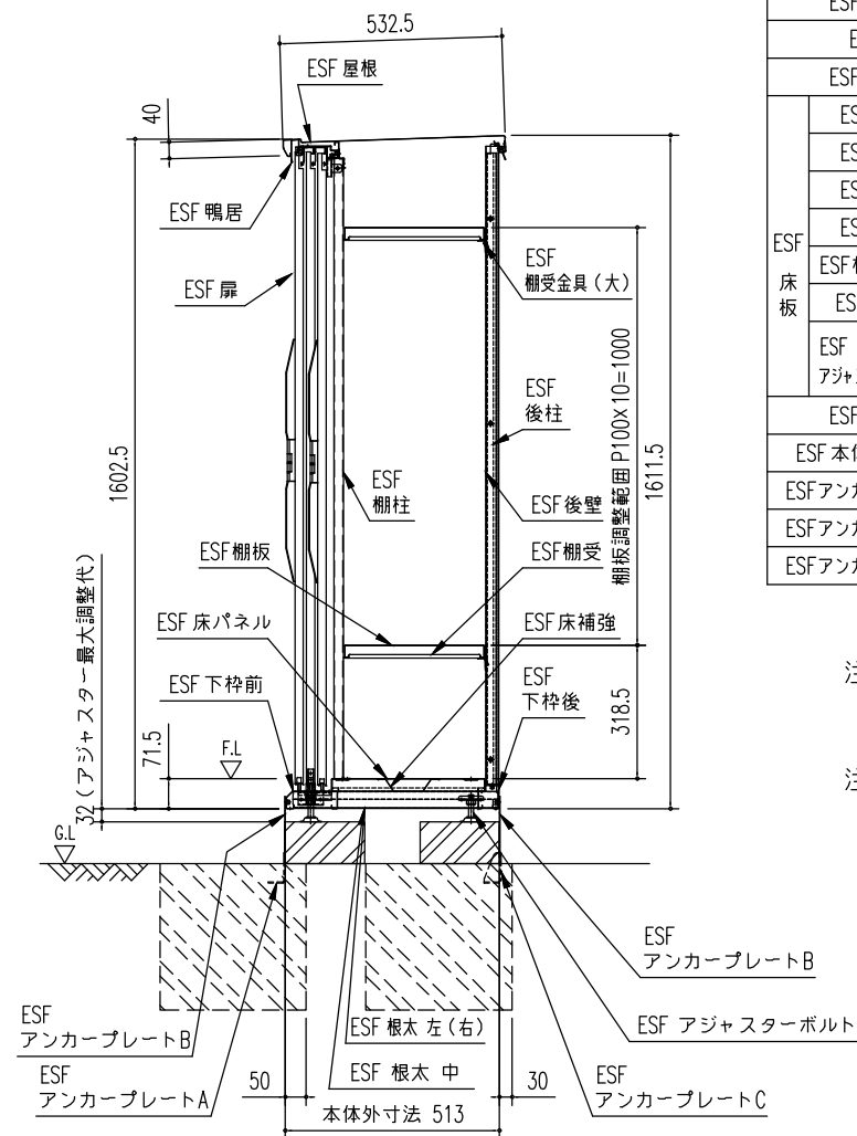
矩計図 (S=1/20)
