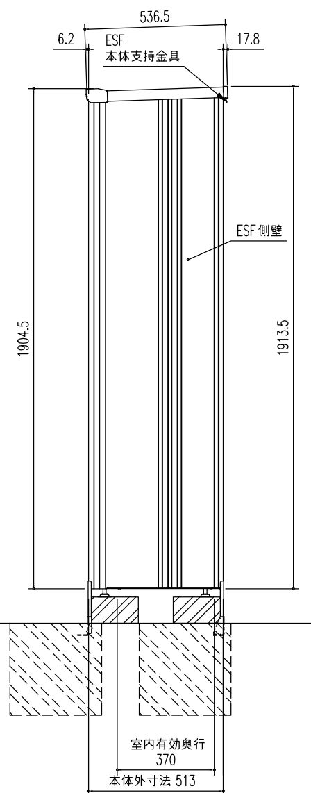
側面図 (S=1/20)
