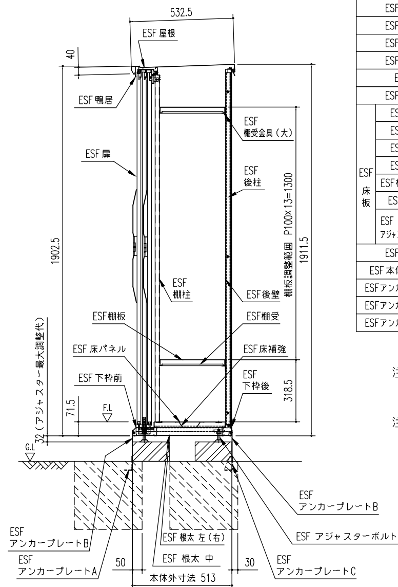
矩計図 (S=1/20)
