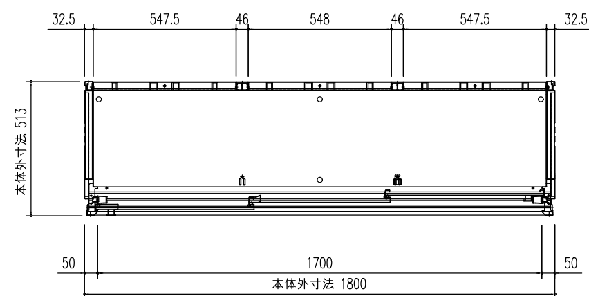
平面図 (S=1/20)
