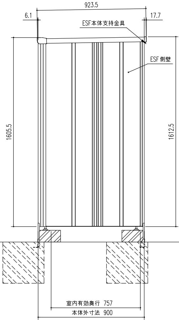
側面図 (S=1/20)
