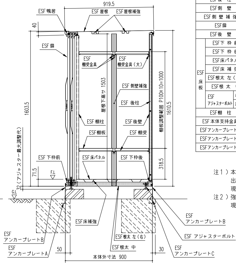
矩計図 (S=1/20)
