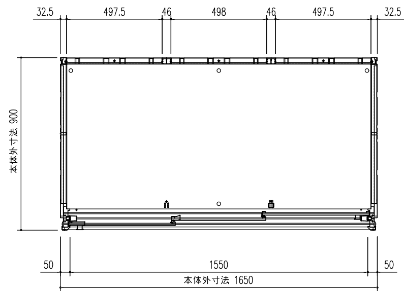
平面図 (S=1/20)
