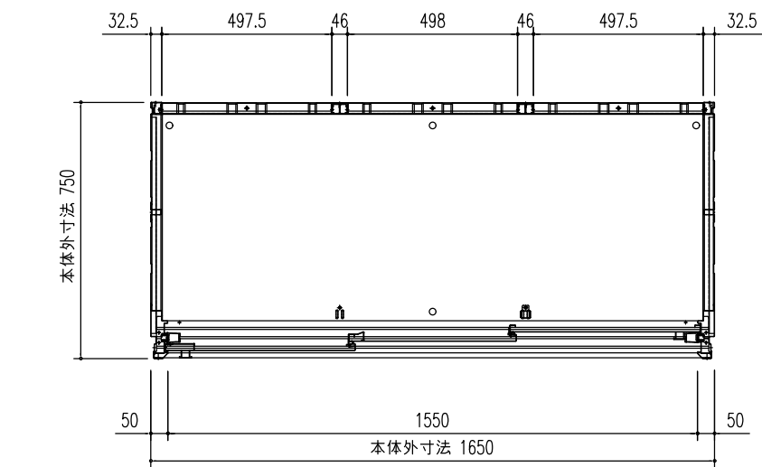
平面図 (S=1/20)
