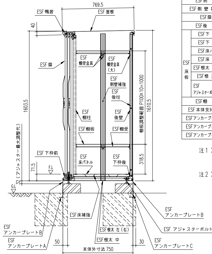
矩計図 (S=1/20)
