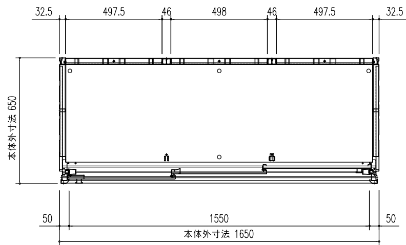
平面図 (S=1/20)
