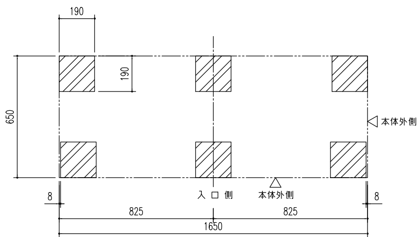
ブロック基礎伏図 (S=1/20)
