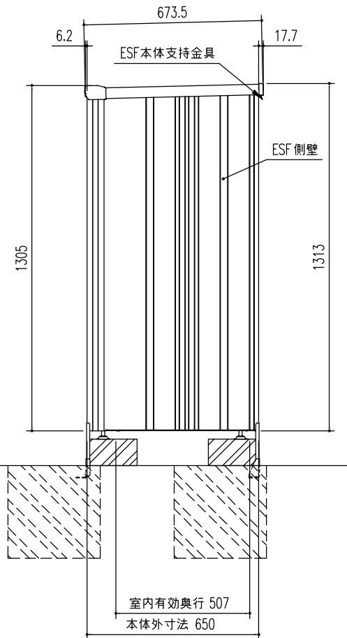
側面図 (S=1/20)
