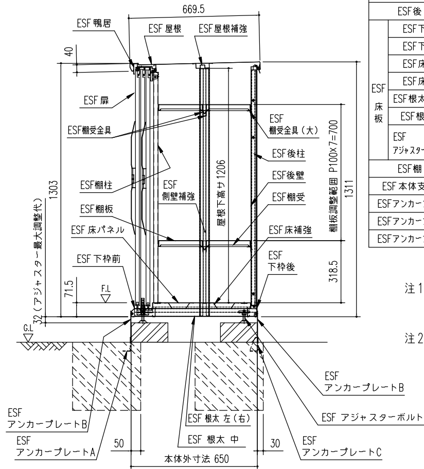
矩計図 (S=1/20)
