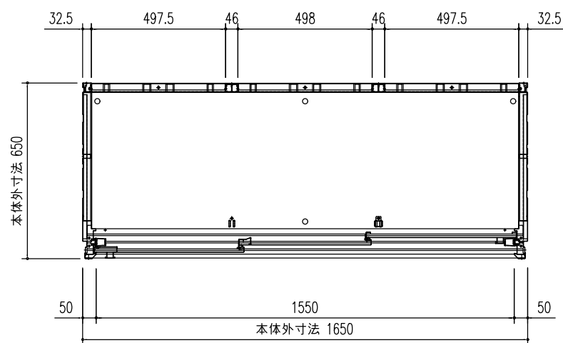
平面図 (S=1/20)
