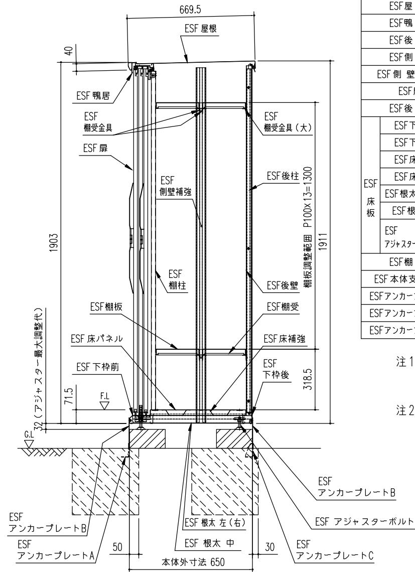
矩計図 (S=1/20)
