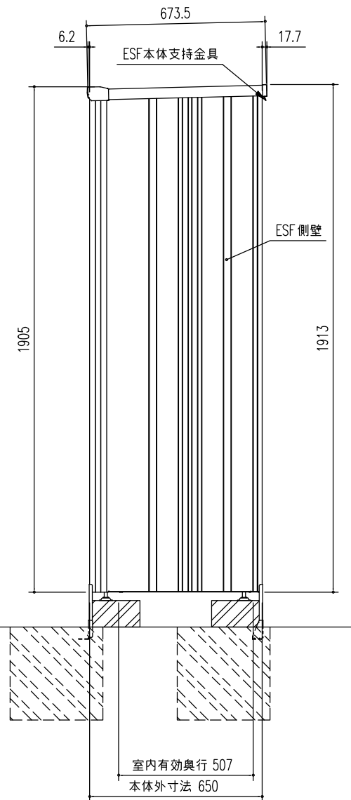
側面図 (S=1/20)
