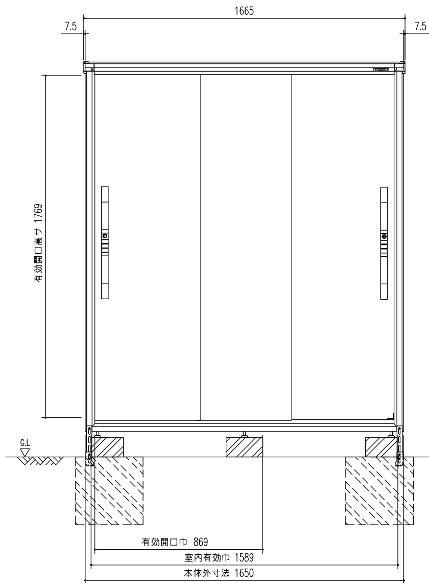
正面立面図 (S=1/20)
