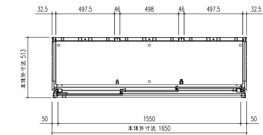
平面図 (S=1/20)
