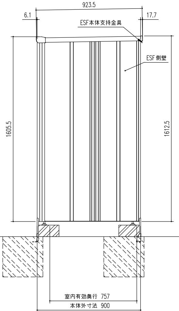
側面図 (S=1/20)
