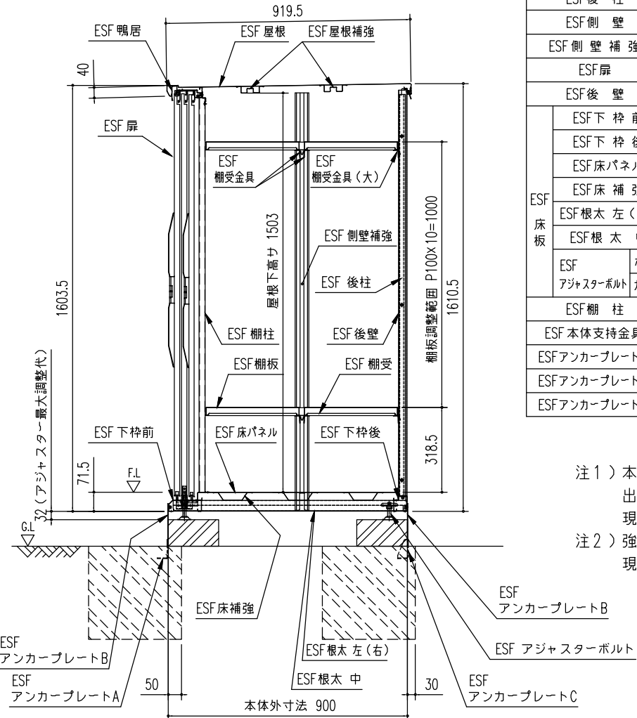
矩計図 (S=1/20)
