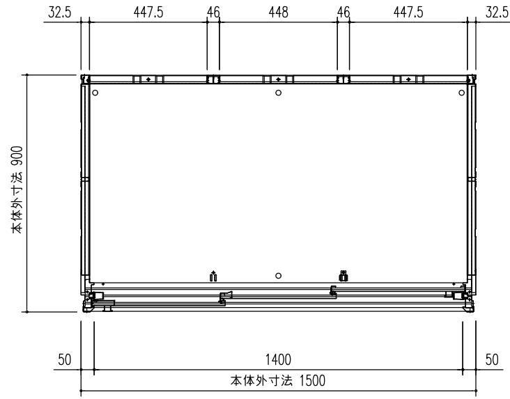
平面図 (S=1/20)
