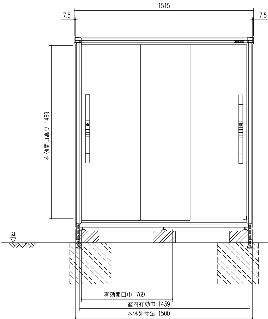
正面立面図 (S=1/20)
