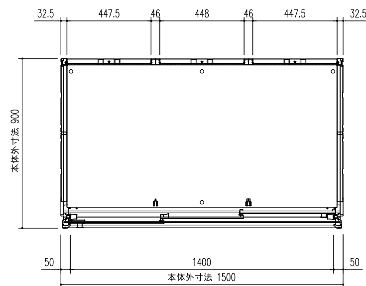
平面図 (S=1/20)
