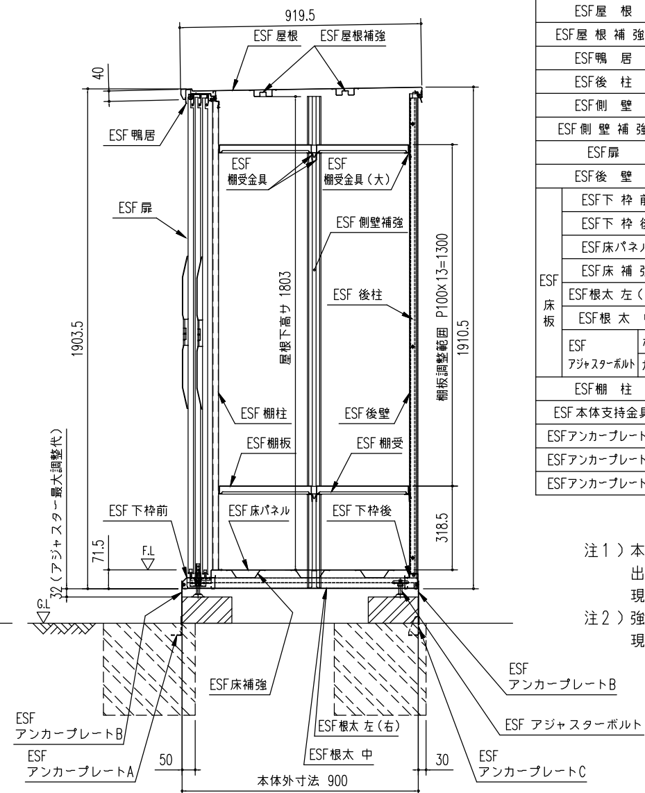
矩 計 図 (S=1/20)
