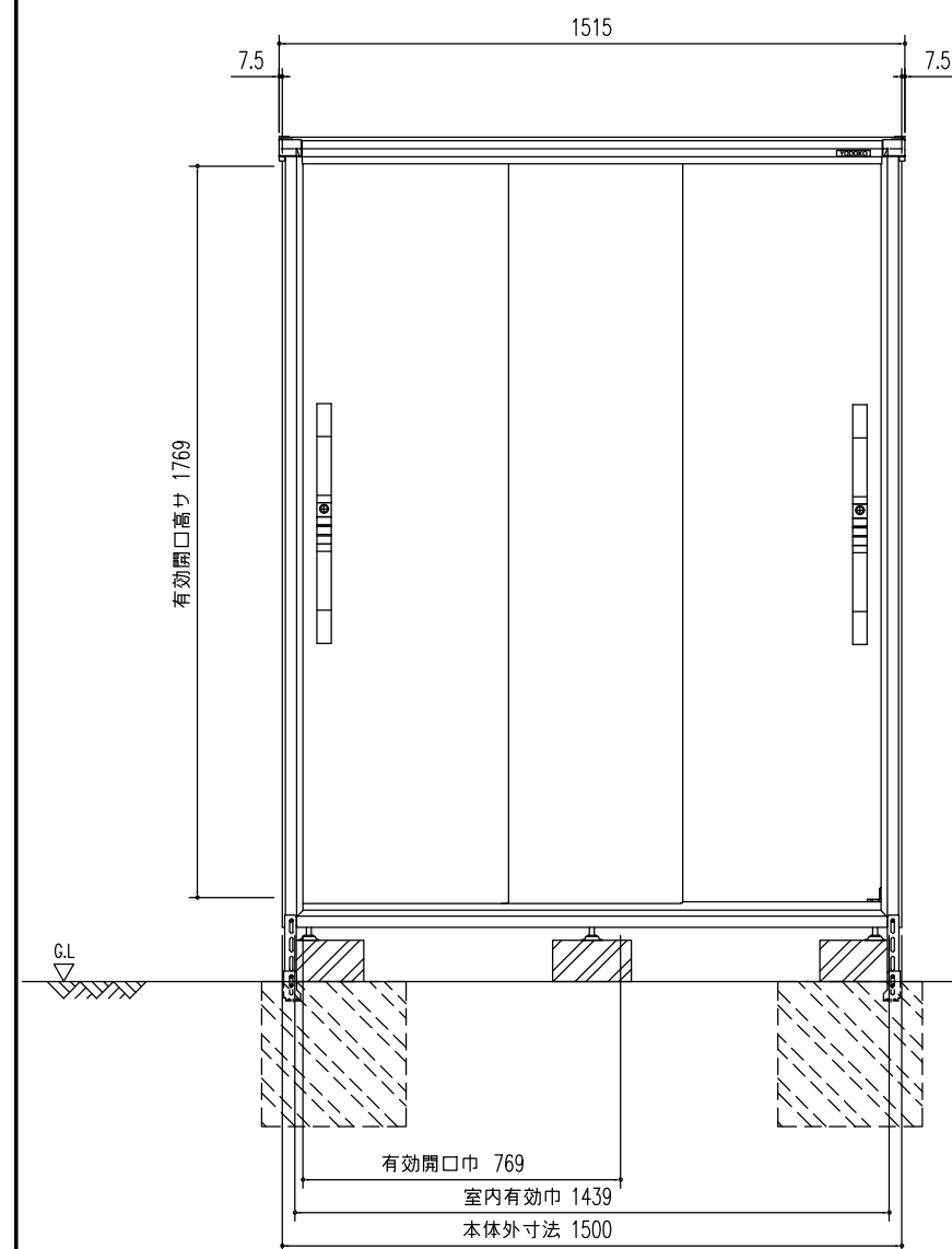
正面立面图 (S=1/20)
