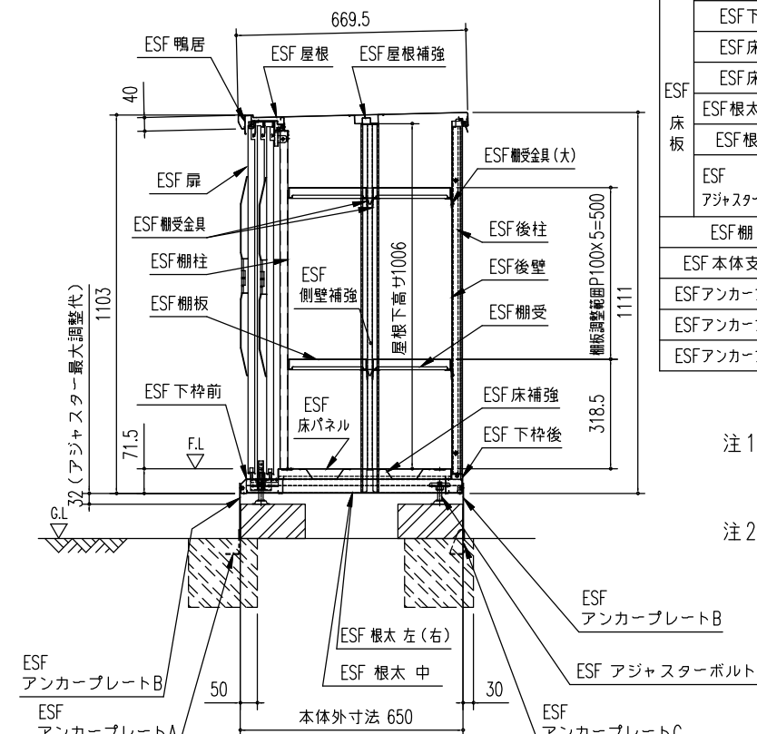
矩 計 図 (S=1/20)
