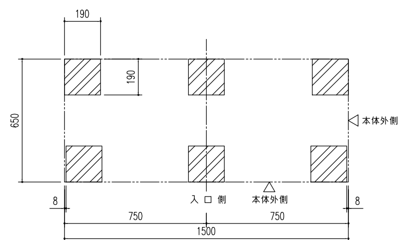
ブロック基礎伏図 (S=1/20)
