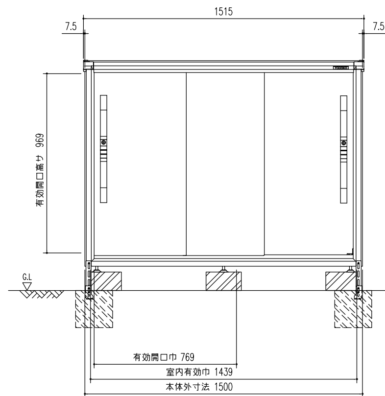
正面立面图 (S=1/20)
