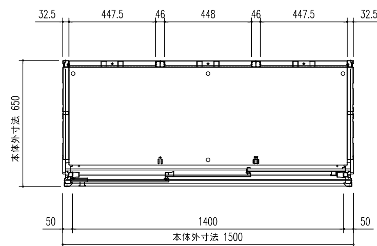
平面図 (S=1/20)
