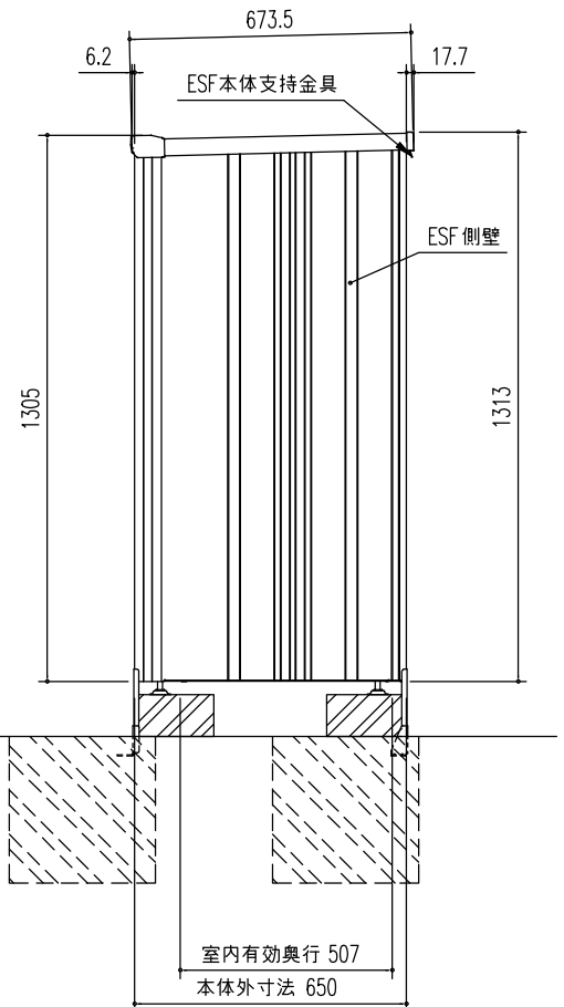
側面図 (S=1/20)
