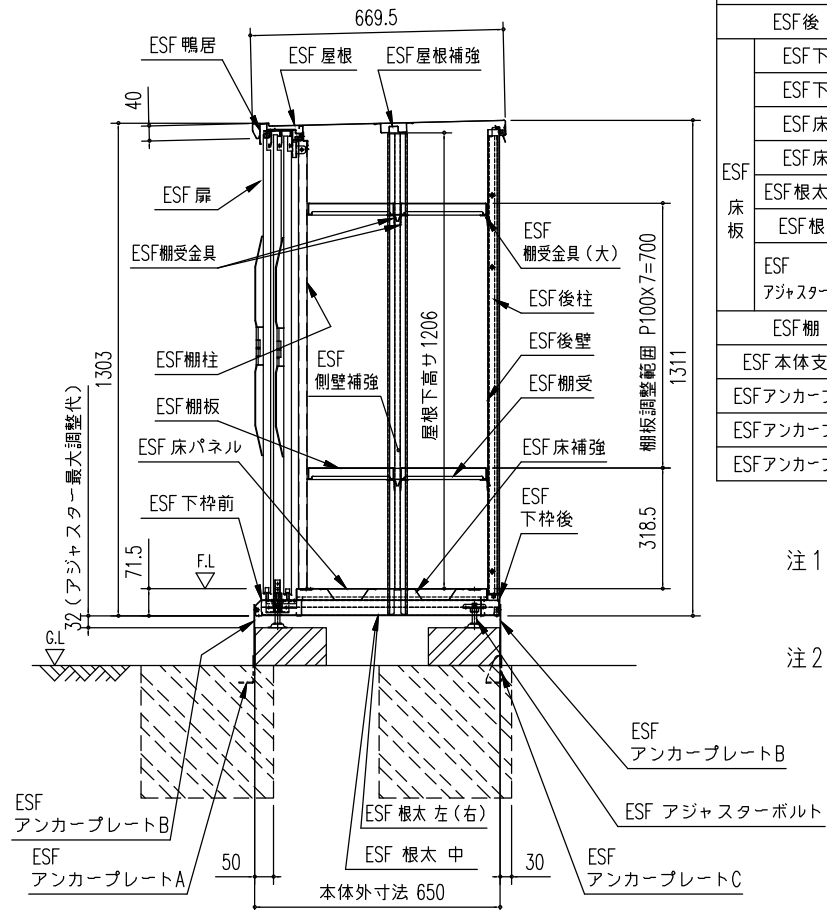
矩計図 (S=1/20)
