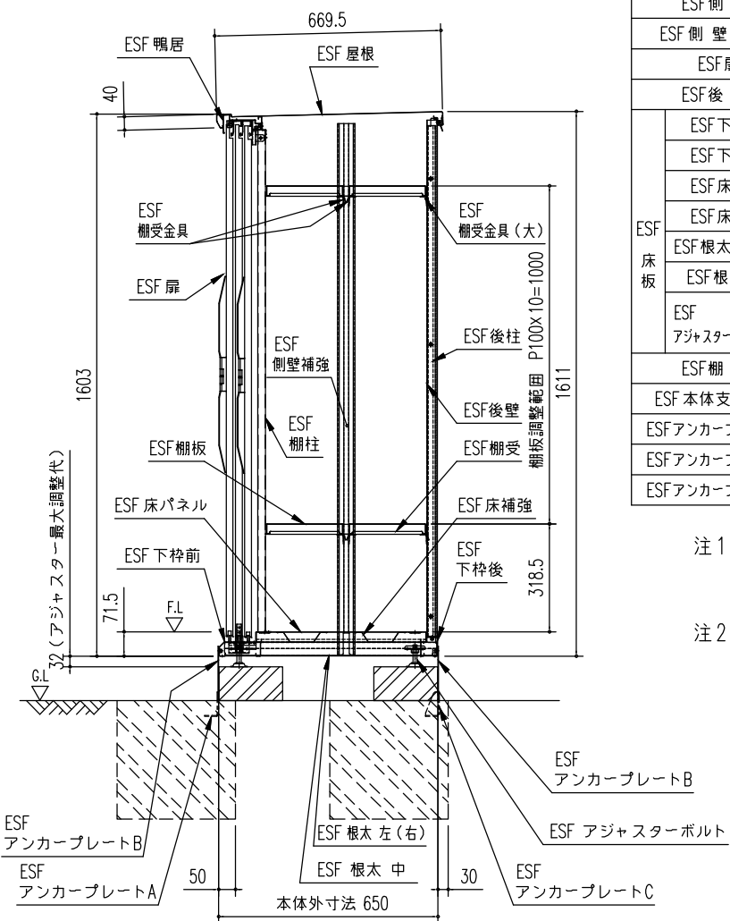
矩計図 (S=1/20)
