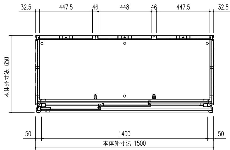
平面図 (S=1/20)
