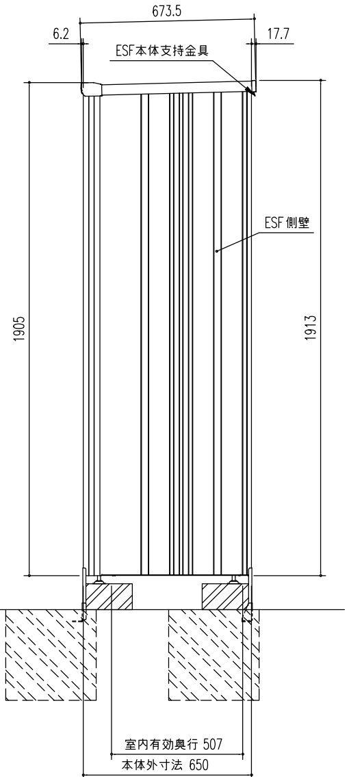
側面図 (S=1/20)
