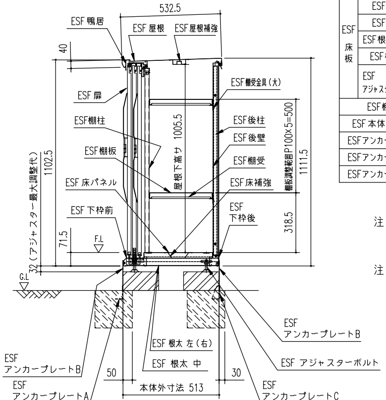
矩計図 (S=1/20)
