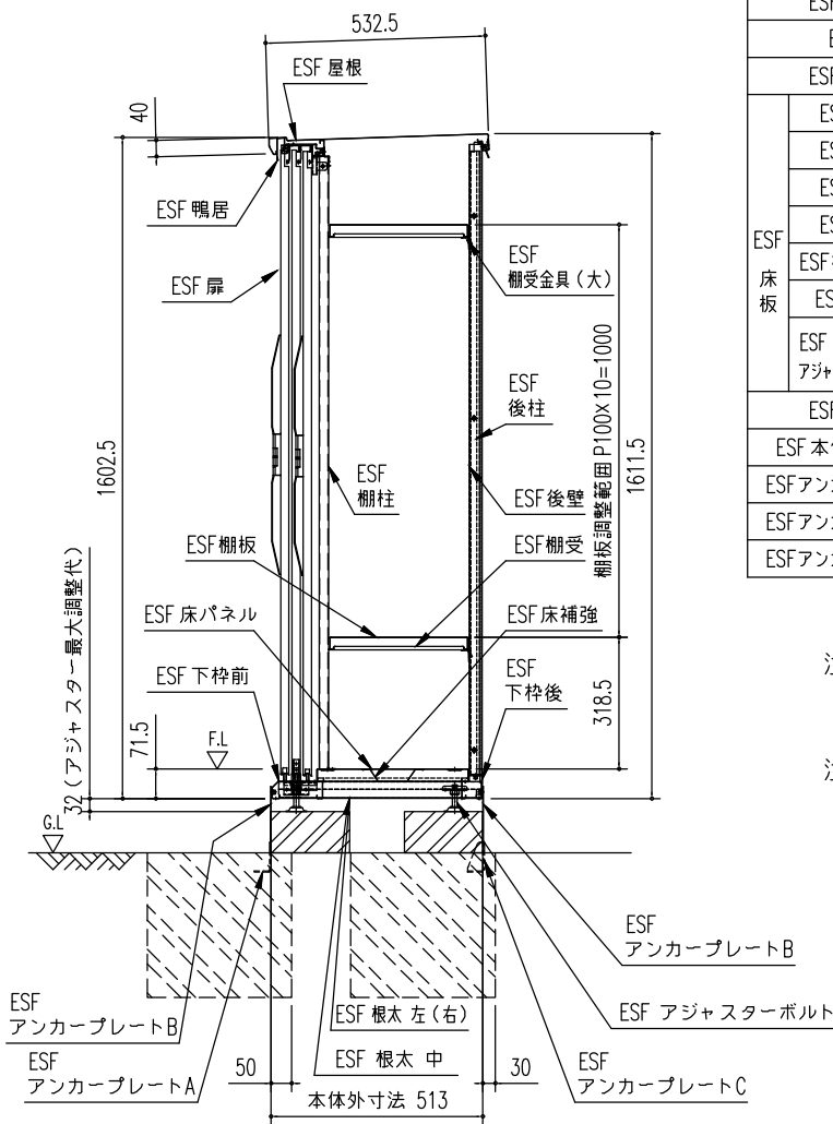
矩計図 (S=1/20)
