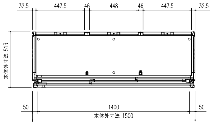
平面図 (S=1/20)
