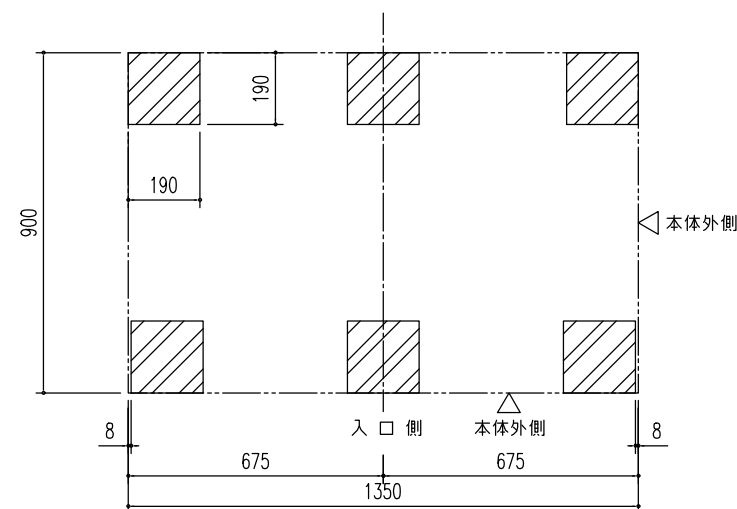
ブロック基礎伏図 (S=1/20)
