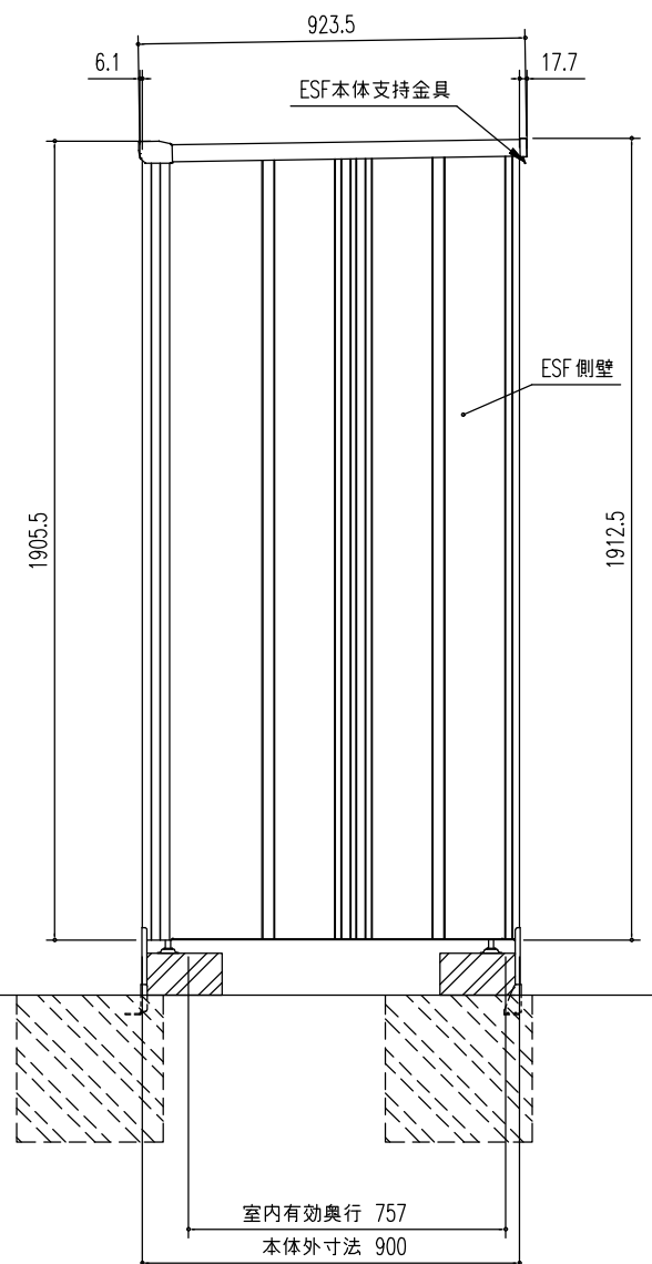
側 面 図 (S=1/20)
