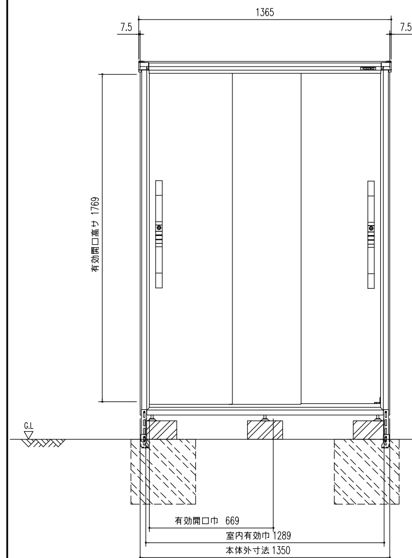
正面立面图 (S=1/20)
