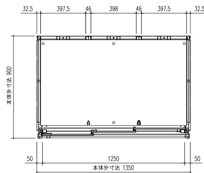
平面図 (S=1/20)
