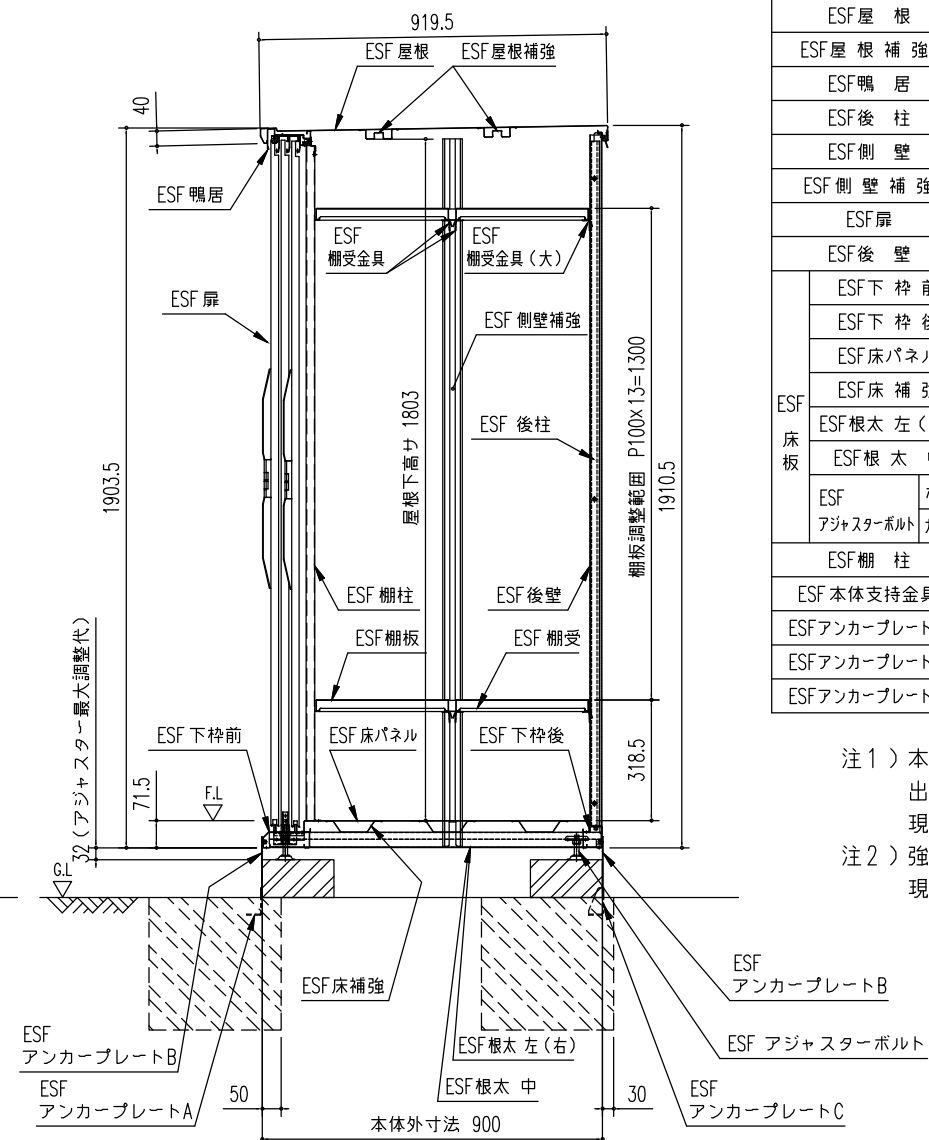
矩 計 図 (S=1/20)
