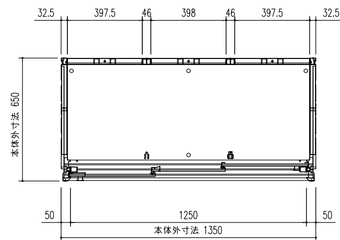
平面図 (S=1/20)
