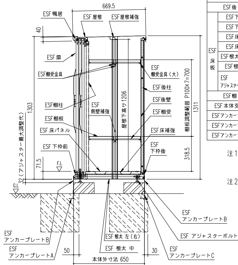
矩計図 (S=1/20)
