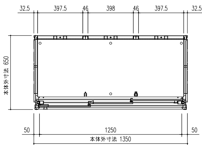
平面図 (S=1/20)
