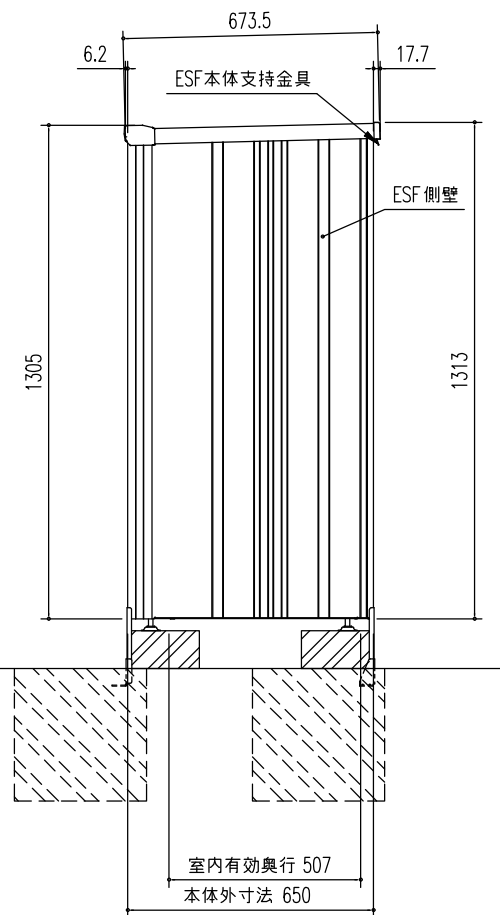
側面図 (S=1/20)
