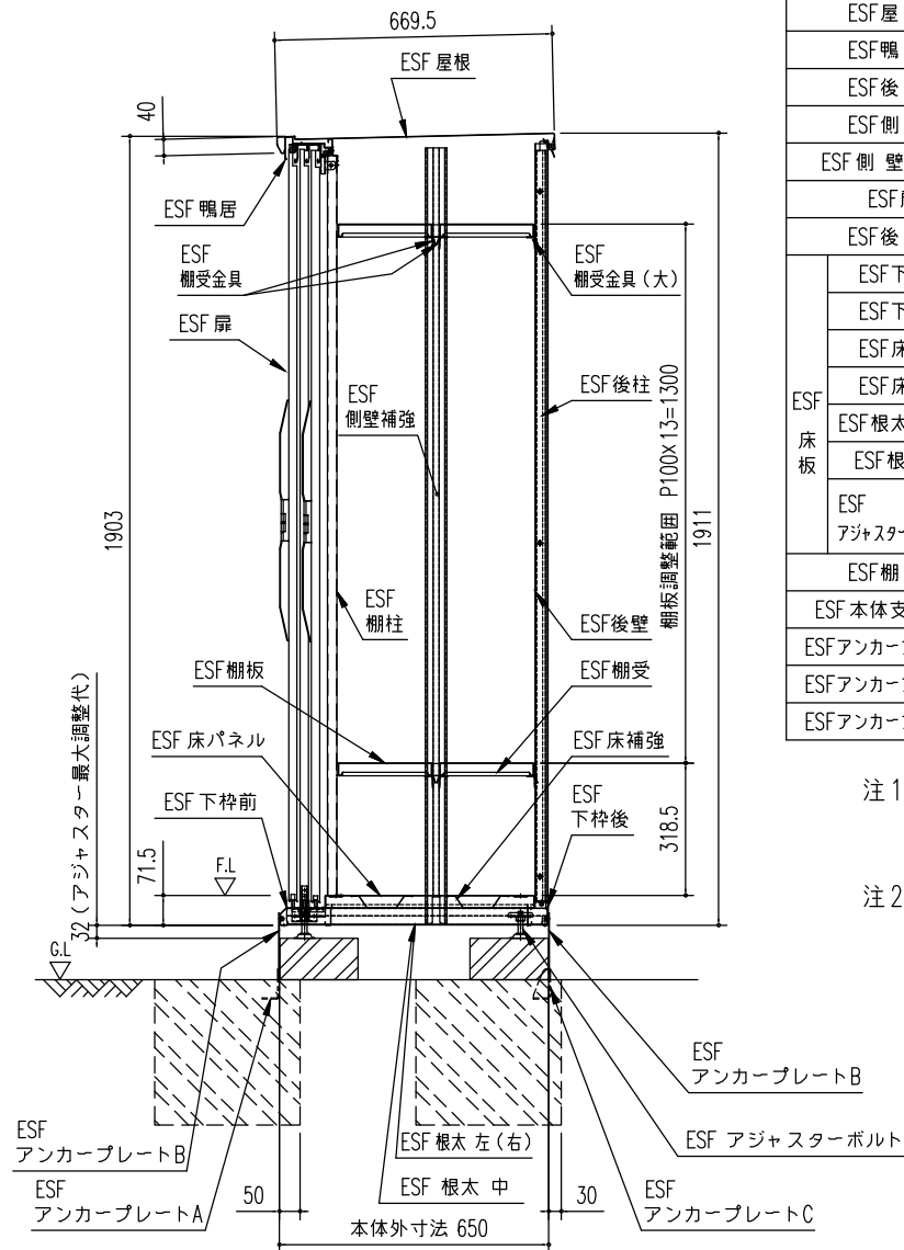
矩計図 (S=1/20)
