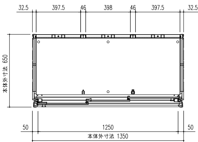
平面図 (S=1/20)
