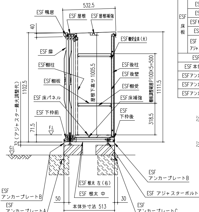
矩計図 (S=1/20)
