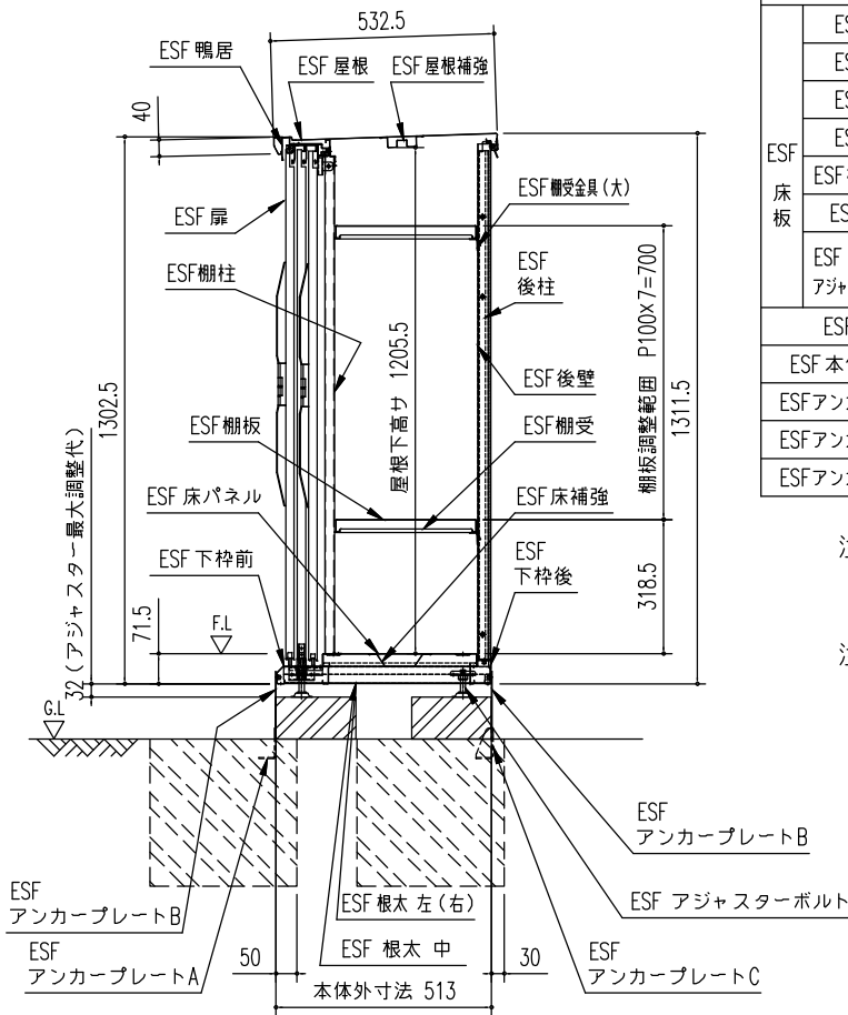
矩計図 (S=1/20)
