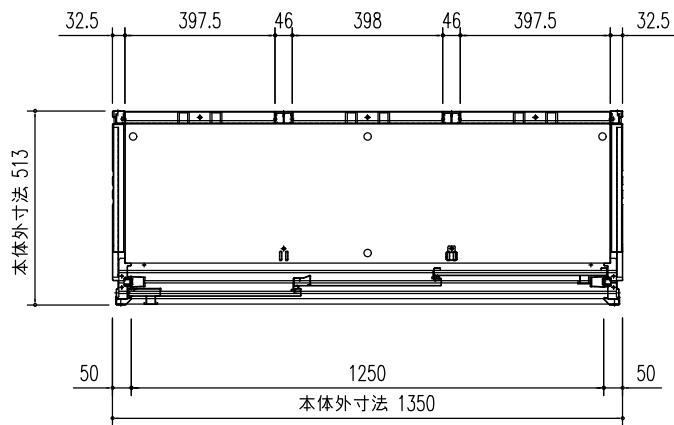
平面図 (S=1/20)
