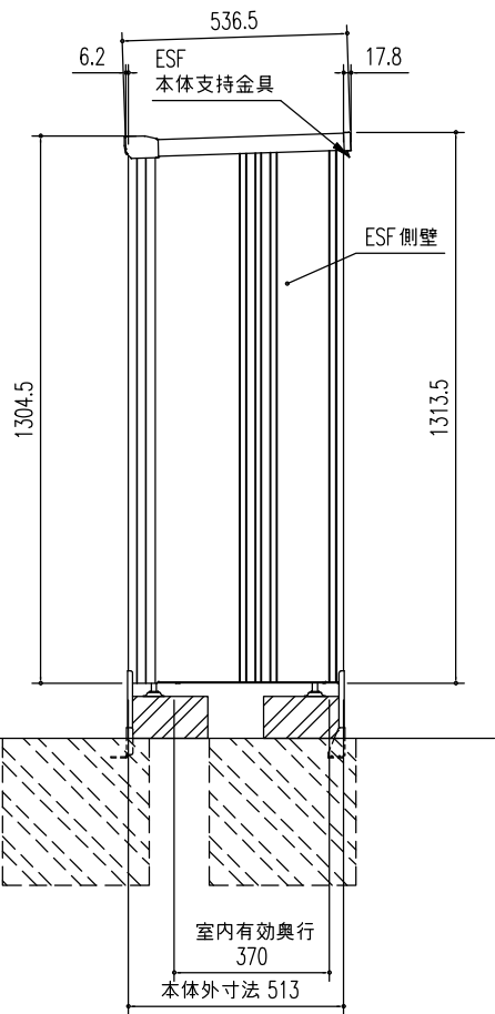
側面図 (S=1/20)
