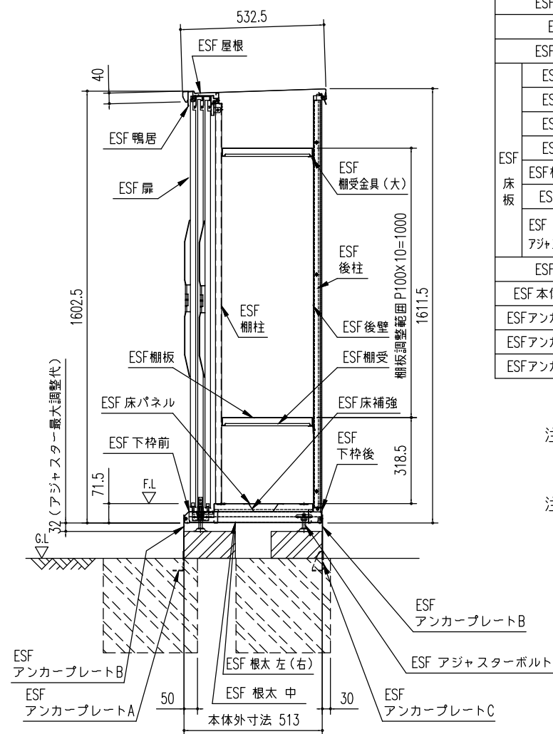
矩計図 (S=1/20)
