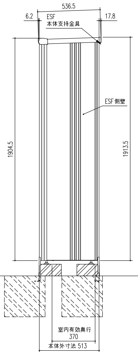
側面図 (S=1/20)
