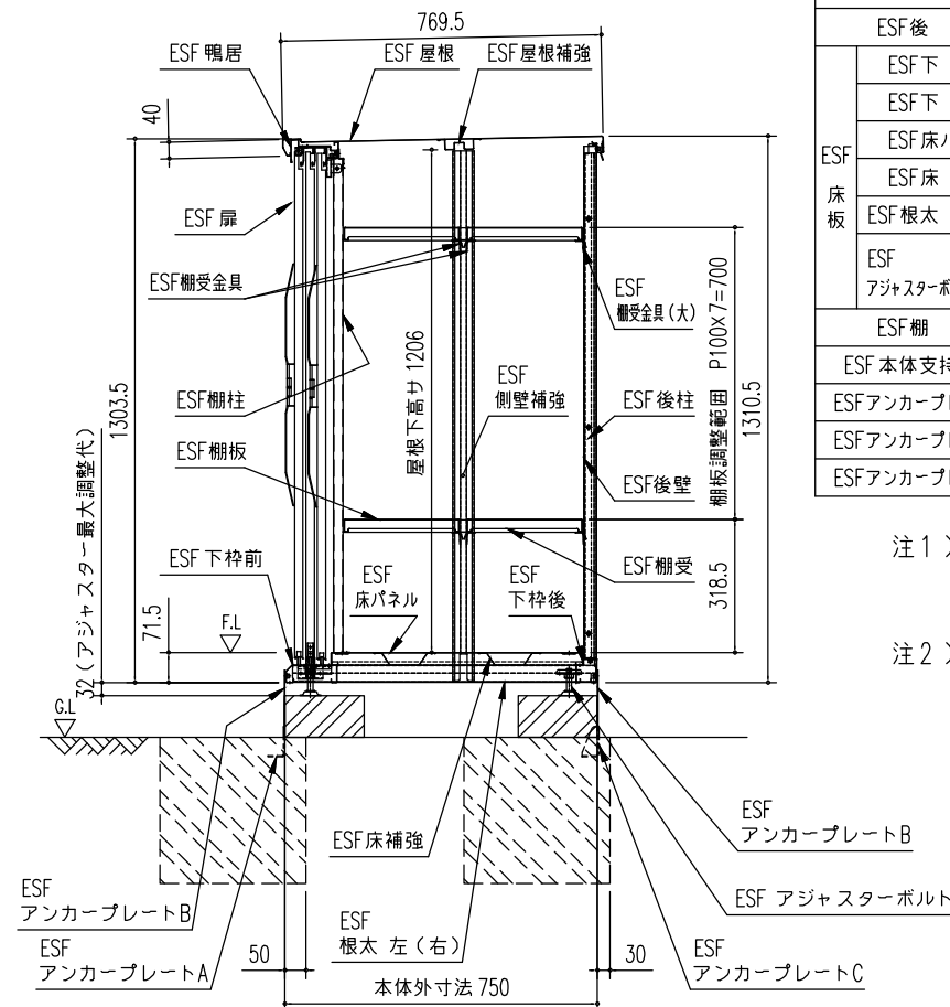
矩計図 (S=1/20)
