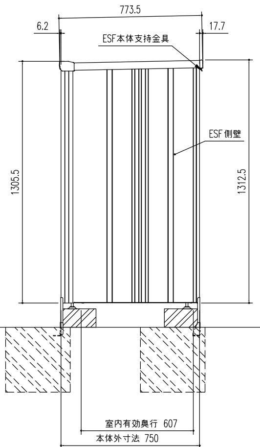
側面図 (S=1/20)
