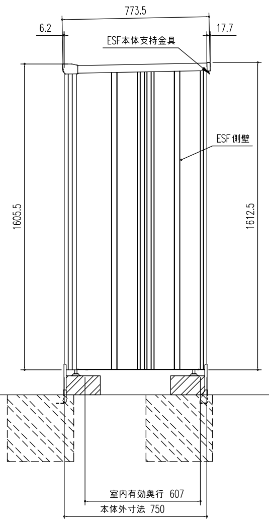
側面図 (S=1/20)
