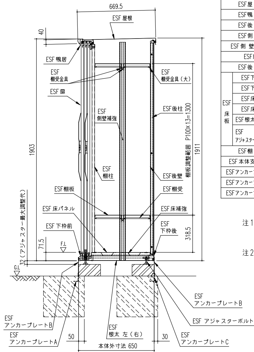
矩計図 (S=1/20)
