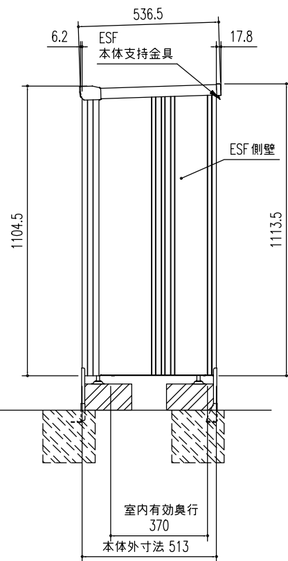
側面図 (S=1/20)
