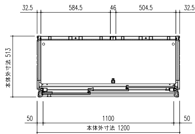
平面図 (S=1/20)
