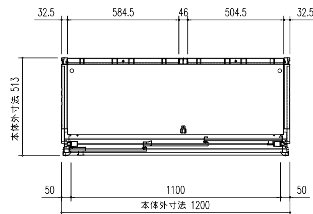
平面図 (S=1/20)
