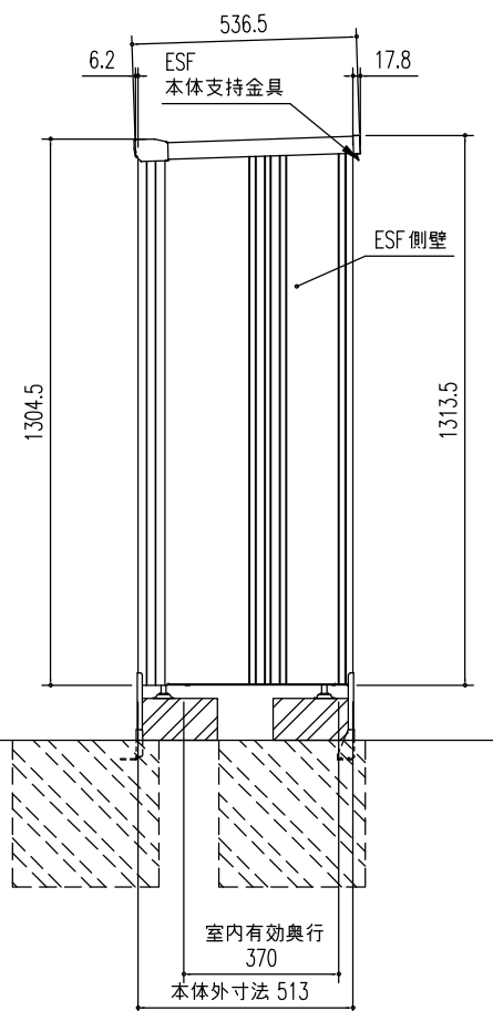
側面図 (S=1/20)
