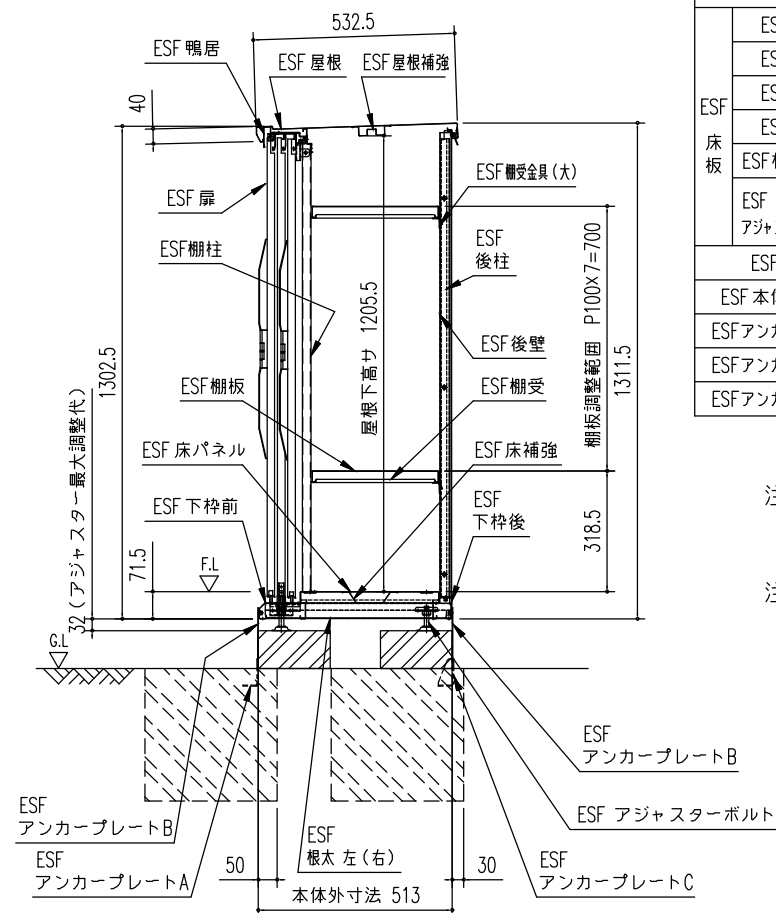
矩計図 (S=1/20)
