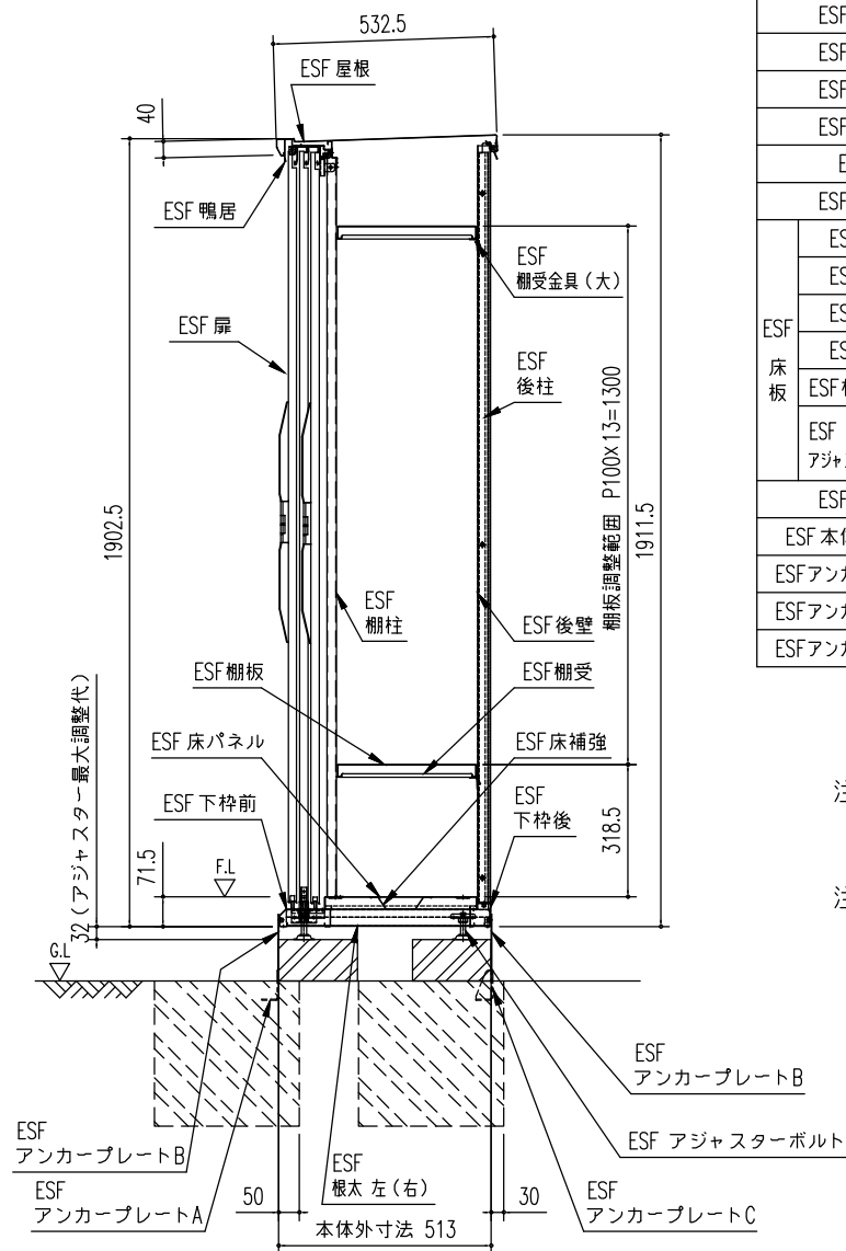
矩計図 (S=1/20)
