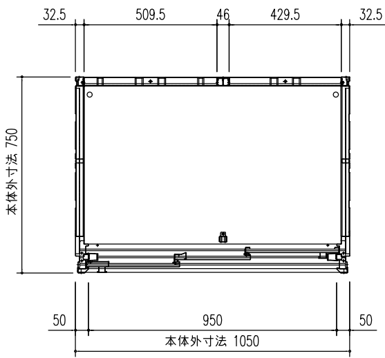
平面図 (S=1/20)
