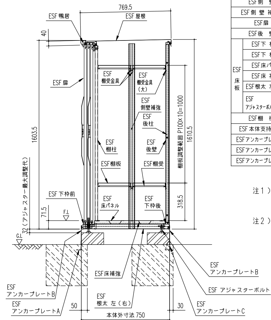
矩 計 図 (S=1/20)
