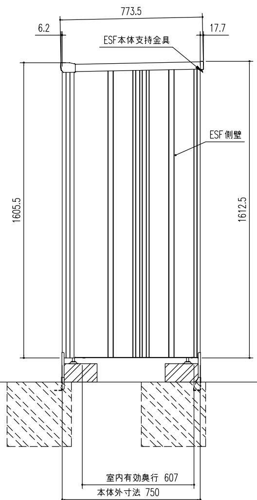
側 面 図 (S=1/20)
