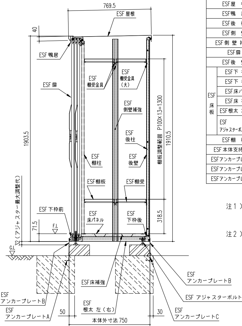
矩計図 (S=1/20)
