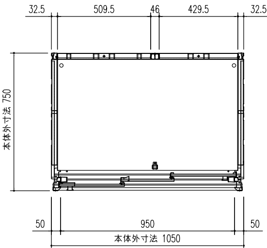
平面図 (S=1/20)
