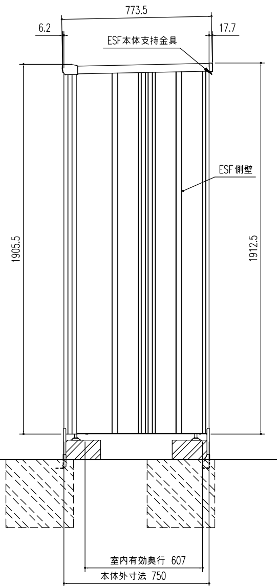
側面図 (S=1/20)
