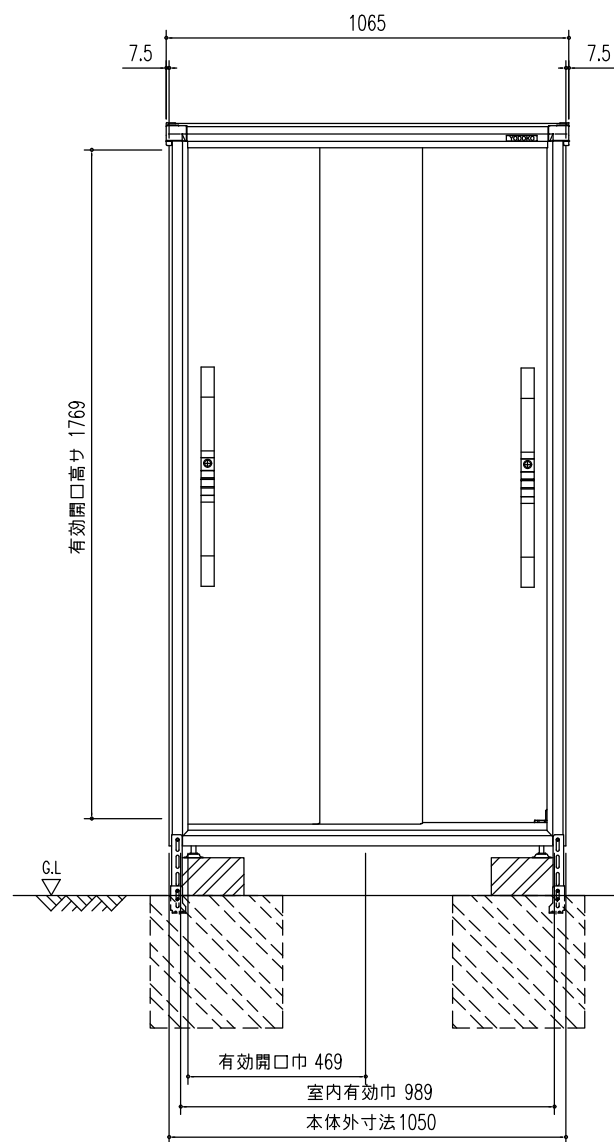
正面立面図 (S=1/20)
