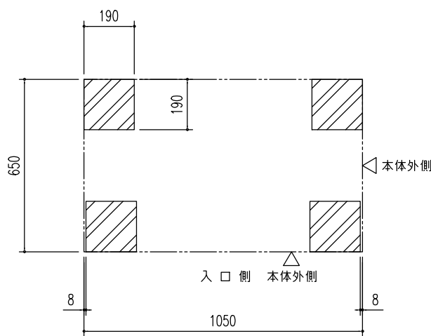
ブロック基礎伏図 (S=1/20)
