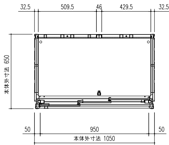
平面図 (S=1/20)
