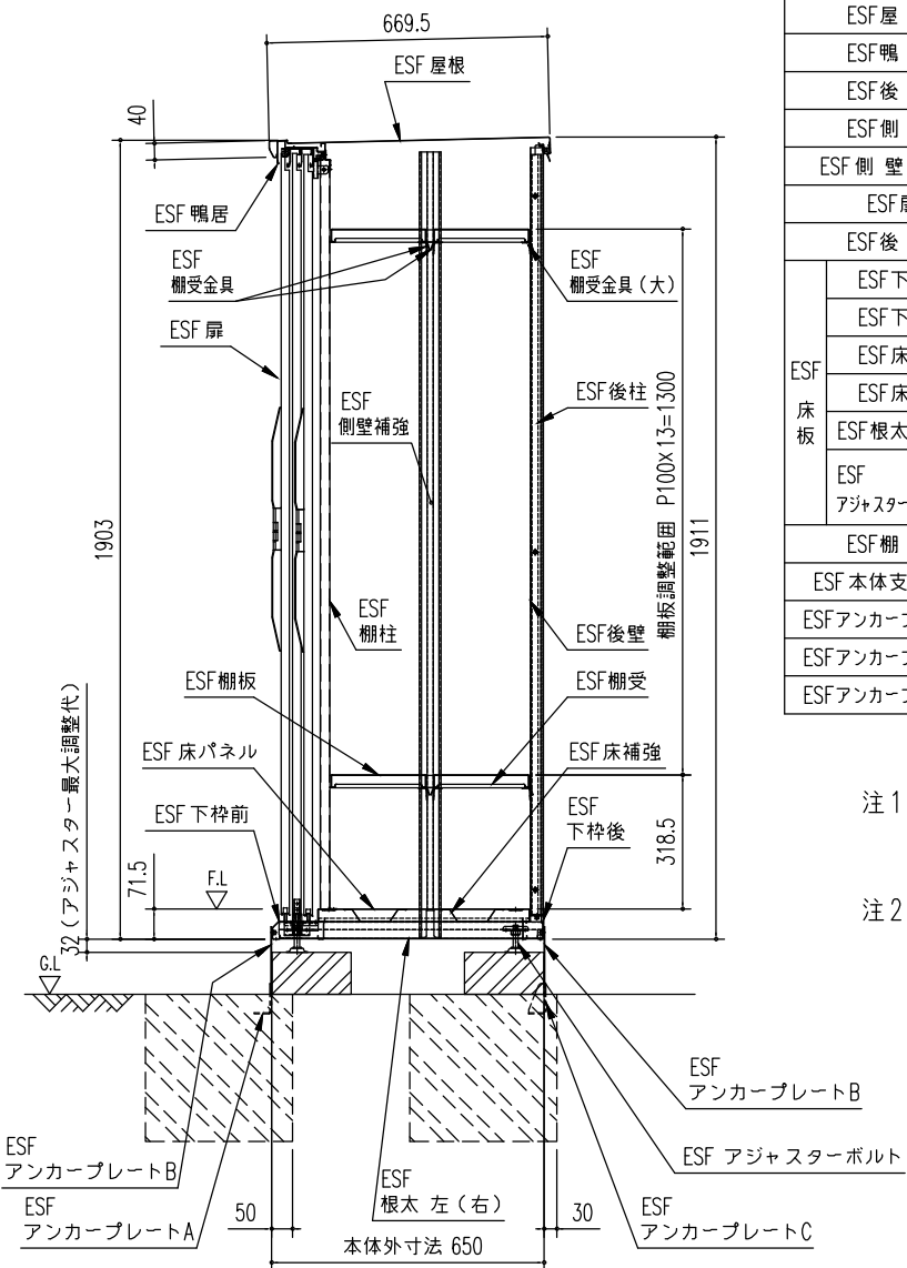
矩計図 (S=1/20)
