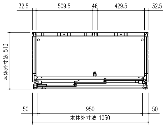
平面図 (S=1/20)
