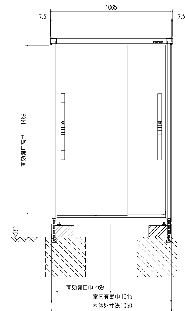
正面立面图 (S=1/20)
