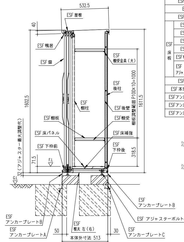
矩 計 図 (S=1/20)
