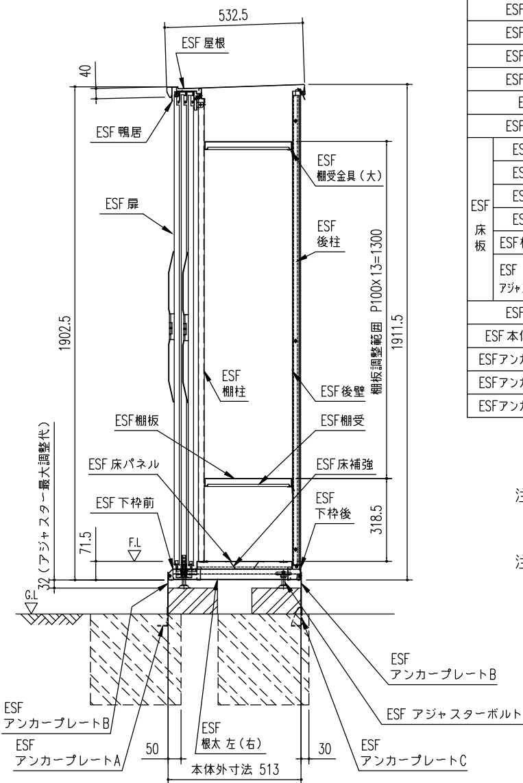
矩計図 (S=1/20)
