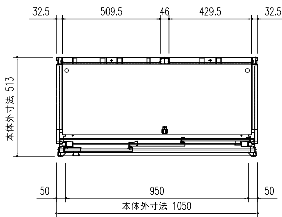
平面図 (S=1/20)
